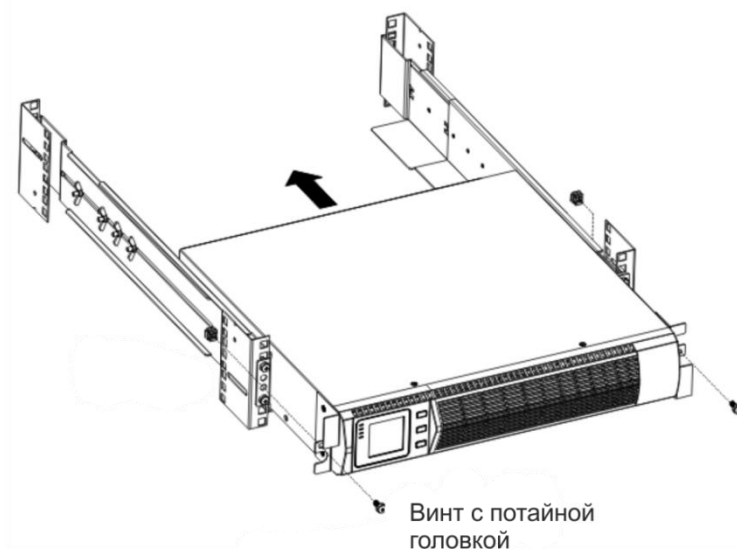
Рисунок 6 – Установка ИБП в стойку
