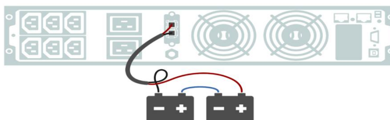
Рисунок 12 – Подключение внешних АКБ к ИБП
