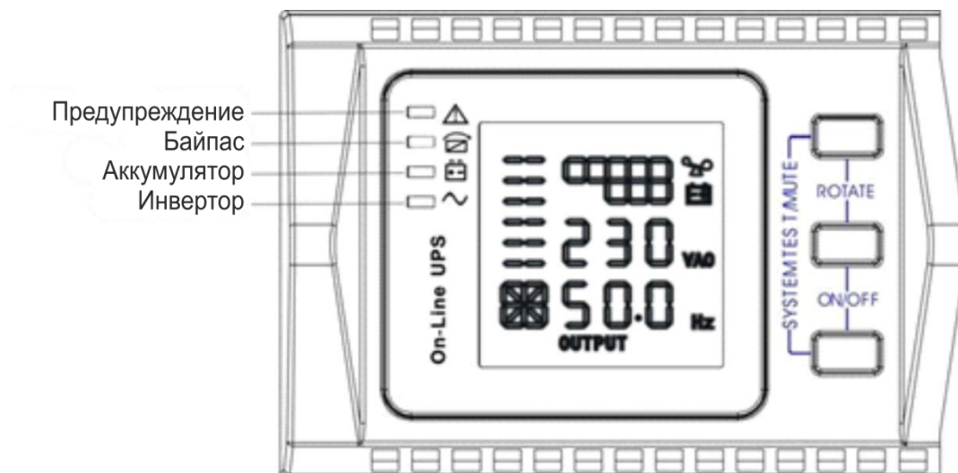
Рисунок 13 – Лицевая панель
