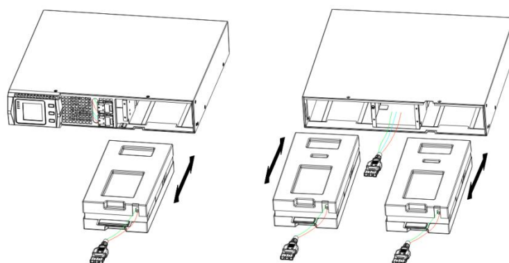
Рисунок 21 – Извлечение блока батарей
