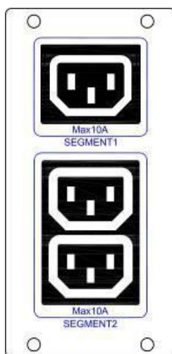
Рисунок 19 – Сегменты нагрузки
