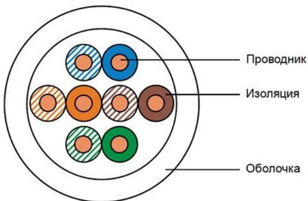
Рисунок 2 - Конструкция кабеля
