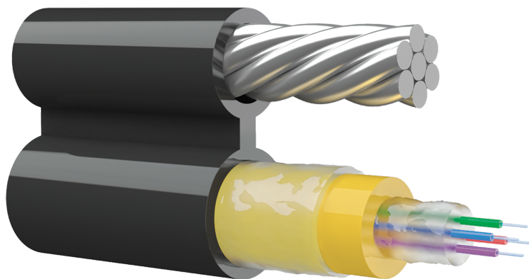
Рисунок 1 - Общий вид
